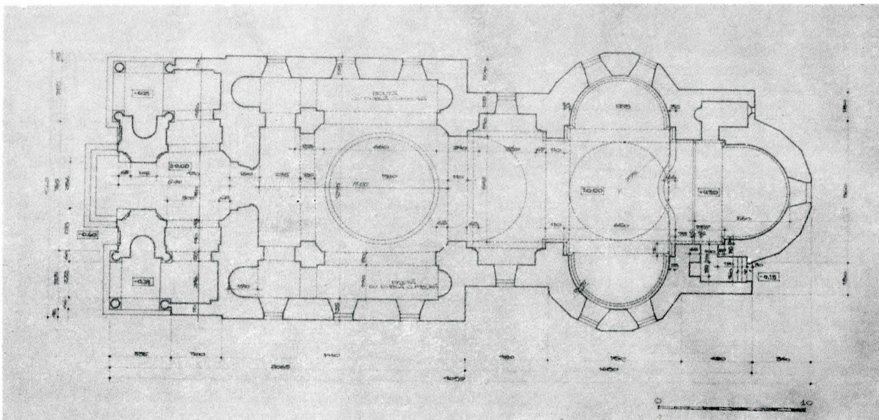
Fig. 3. Plan releveu 1 : 100
