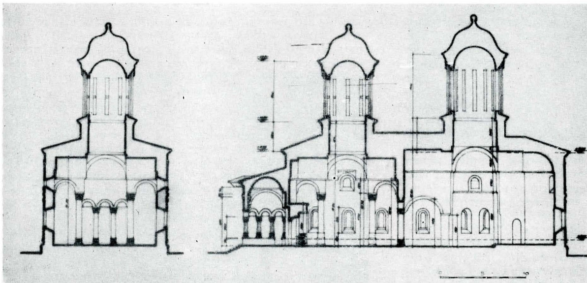
Fig. 5. Secții releveu 1 : 100
